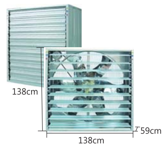
50吋方形負壓扇
