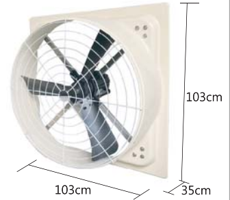
42吋強力循環扇
