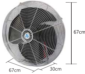
雙圓網
